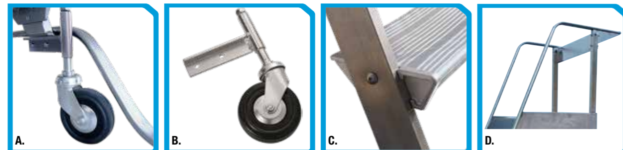
A. Part. attacco e ruota piroettante B. Kit porta ruota scala SG C. Particolare attacco gradino D. Versione con porta oggetti
