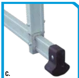
A. Sistema antiapertura scala B. Sistema antisfilo elementi C. Particolare barra stabilizzatrice
